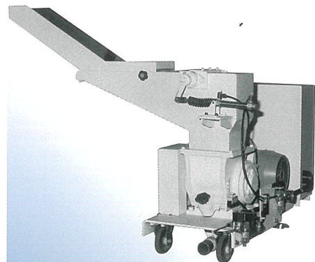
P-1314 投入シュート&エアシリンダ式ダンパ付き 特殊ホッパ・吸引空気輸送タイプ Feed shoot and special hopper with air-cylinder type dumper provided with suction pneumatic transport equipment
