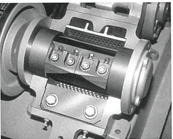
独創的なヘリカルカッタ Unique Helical Cutter
