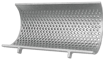
斜穴スクリーン Inclined-hole Screen
