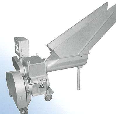
PS-180 特殊投入シュート・自然落下タイプ Special feed shoot (automatic fall type)
