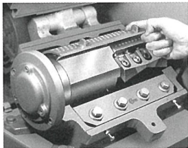
スクリーン交換はワンタッチ 'One touch' replacement of screen
