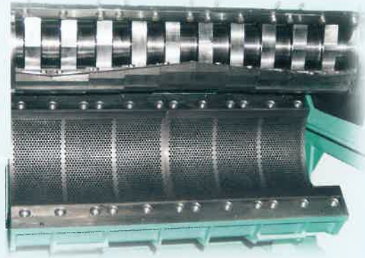
ヘリカルブレード Helical blade
